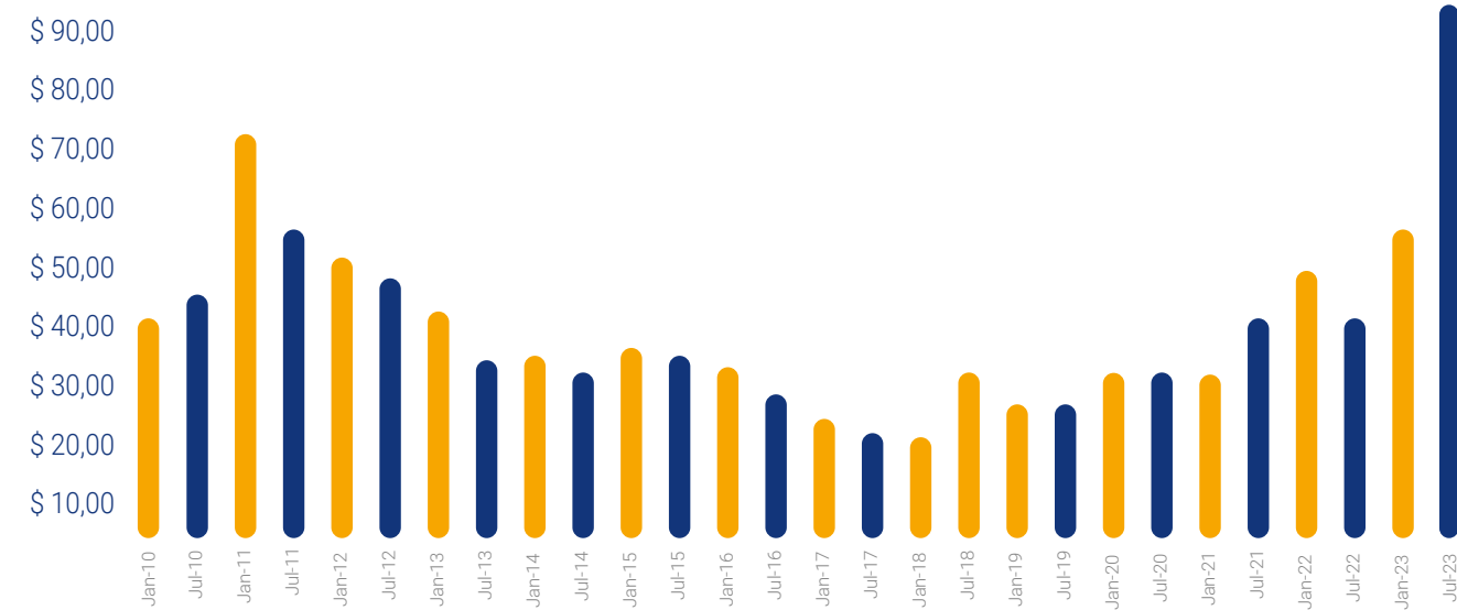
Uranium prices, 2010-2023, USD per lb U 3 O 8 4
